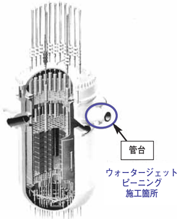
原子炉容器概略図
