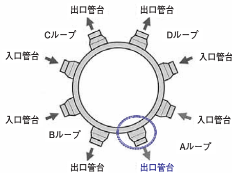
原子炉容器を上から見た概要図
